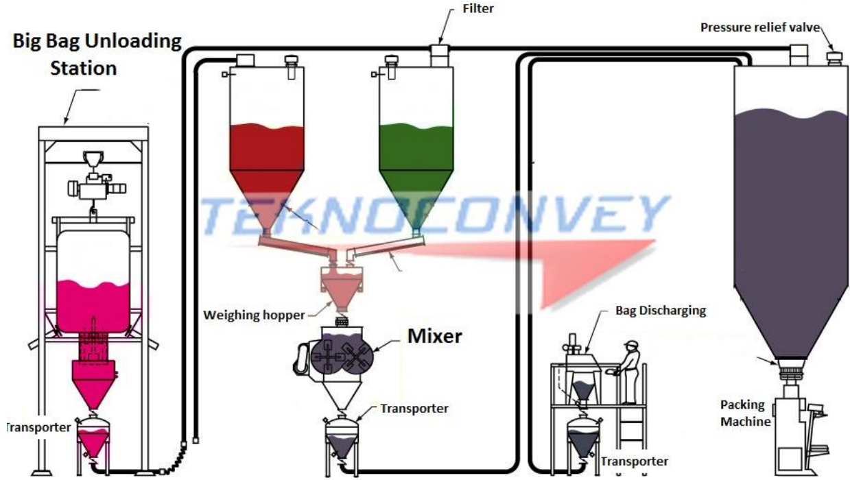
Pnömatik transfer
